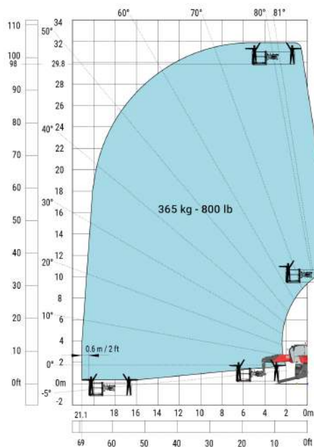
Rotazione su stabilizzatori con cestello da 365 kg
