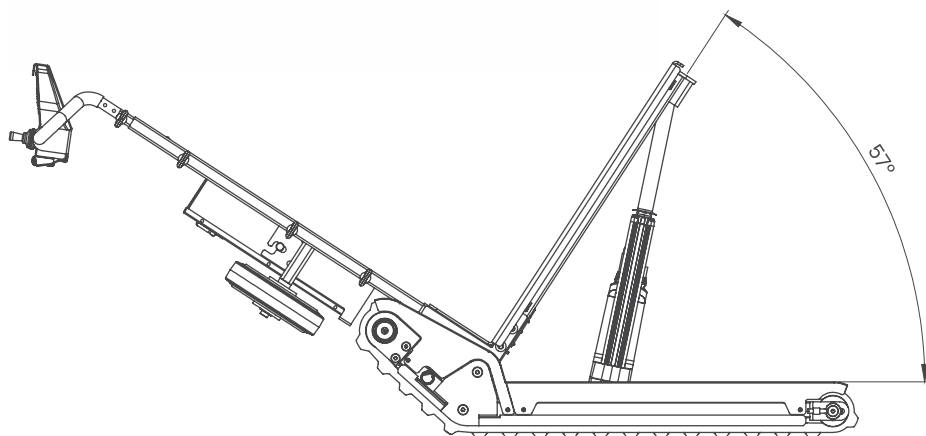
Posizione massima inclinazione piano di carico
