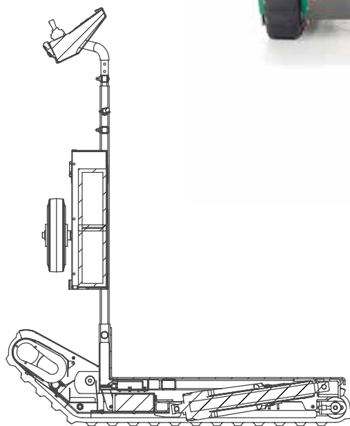
Sezione A-A
